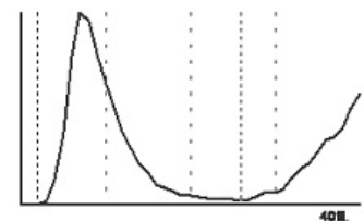
PLT
